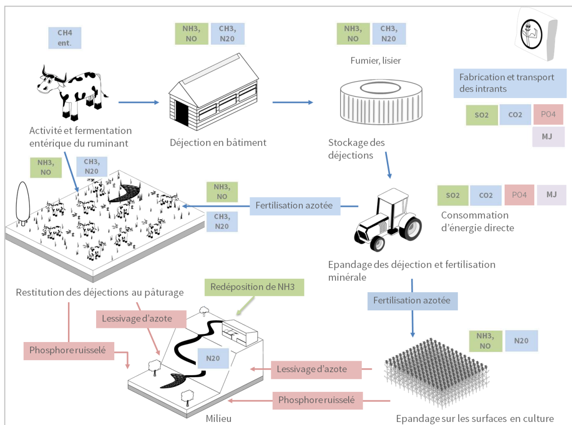
Emissions polluantes le long du cycle de vie de la production laitière agricole
